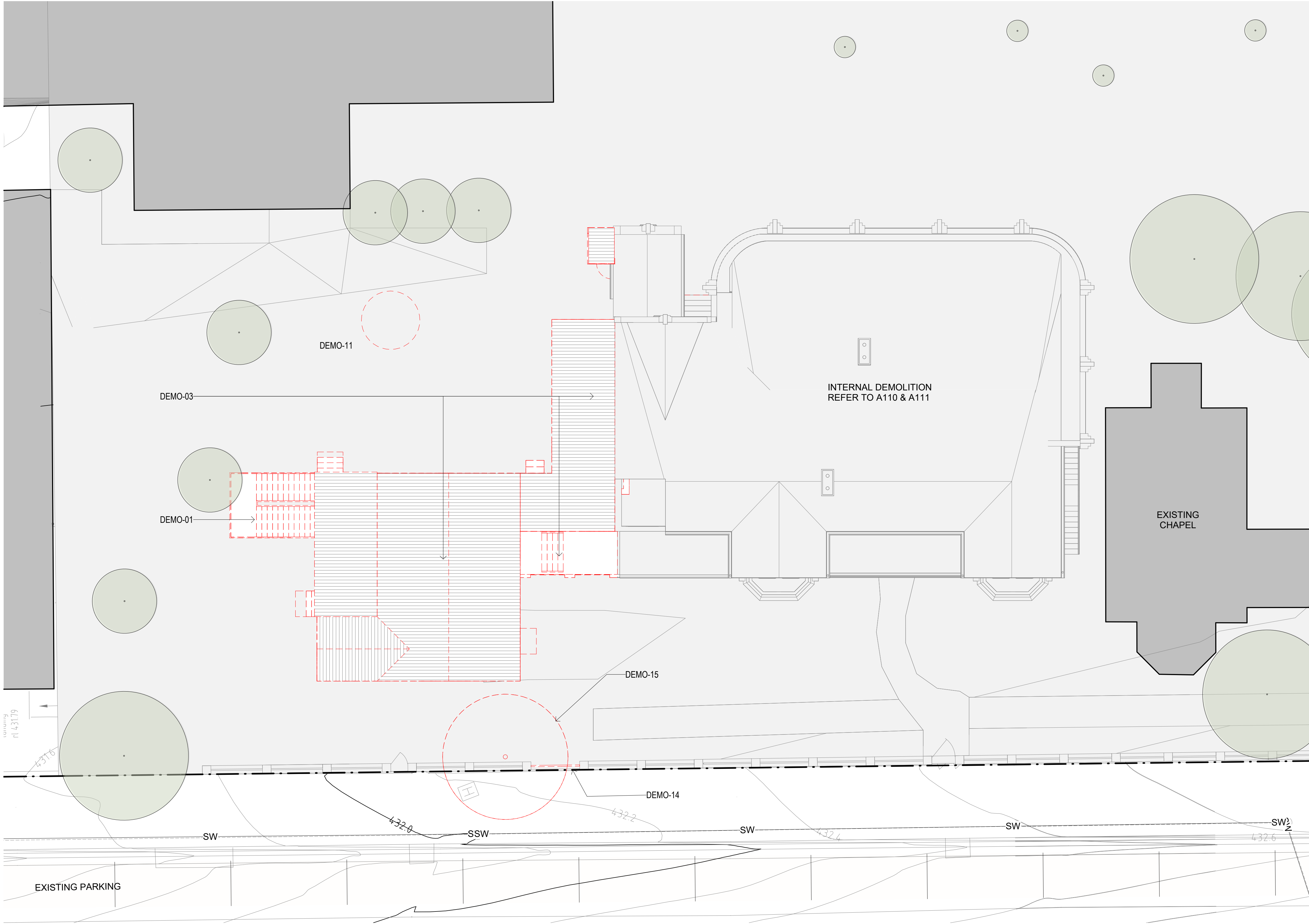
1 SITE - DEMOLITION PLAN A205 1 : 100
